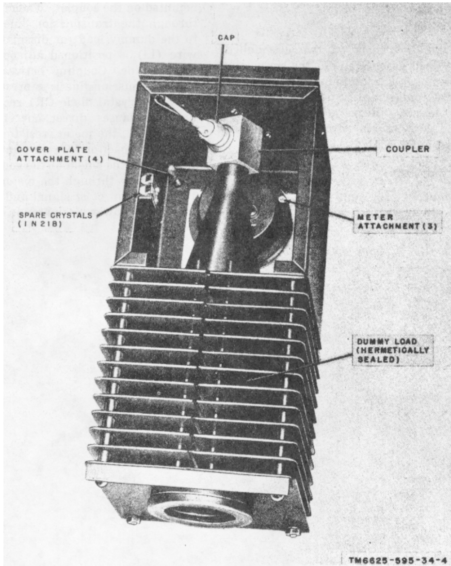
Figure 3-1. Wattmeter ME-82/U, bottom A.
